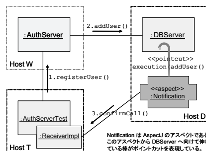
図 1 AspectJ で記述したテストコード Fig. 1 The testing code in AspectJ
