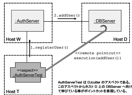
図 2 DJcutter を利用したテストコード Fig.2 The testing code in DJcutter
